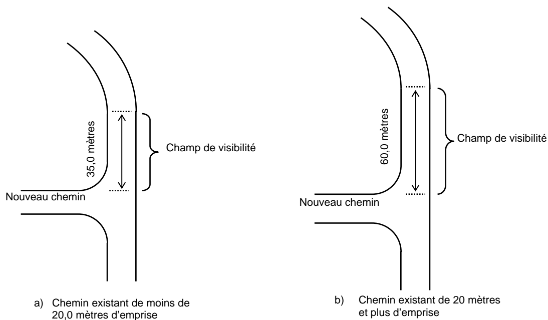
FIGURE 5.5 : CHAMP DE VISIBILITÉ
