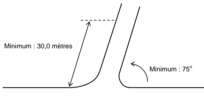
FIGURE 5.4 : ANGLE ENTRE DEUX INTERSECTIONS
