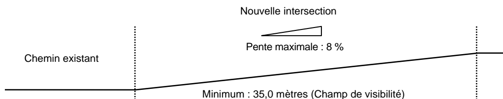
FIGURE 5.6 : PENTE MAXIMALE D'UNE NOUVELLE INTERSECTION
