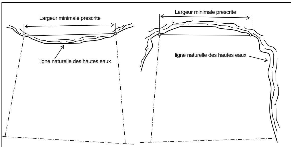
FIGURE 3.3 : LARGEUR MINIMALE D'UN LOT RIVERAIN
