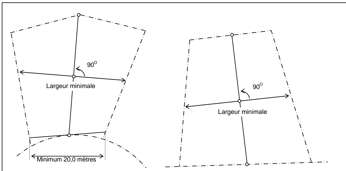
FIGURE 3.3 : LARGEUR MINIMALE D'UN LOT RIVERAIN
