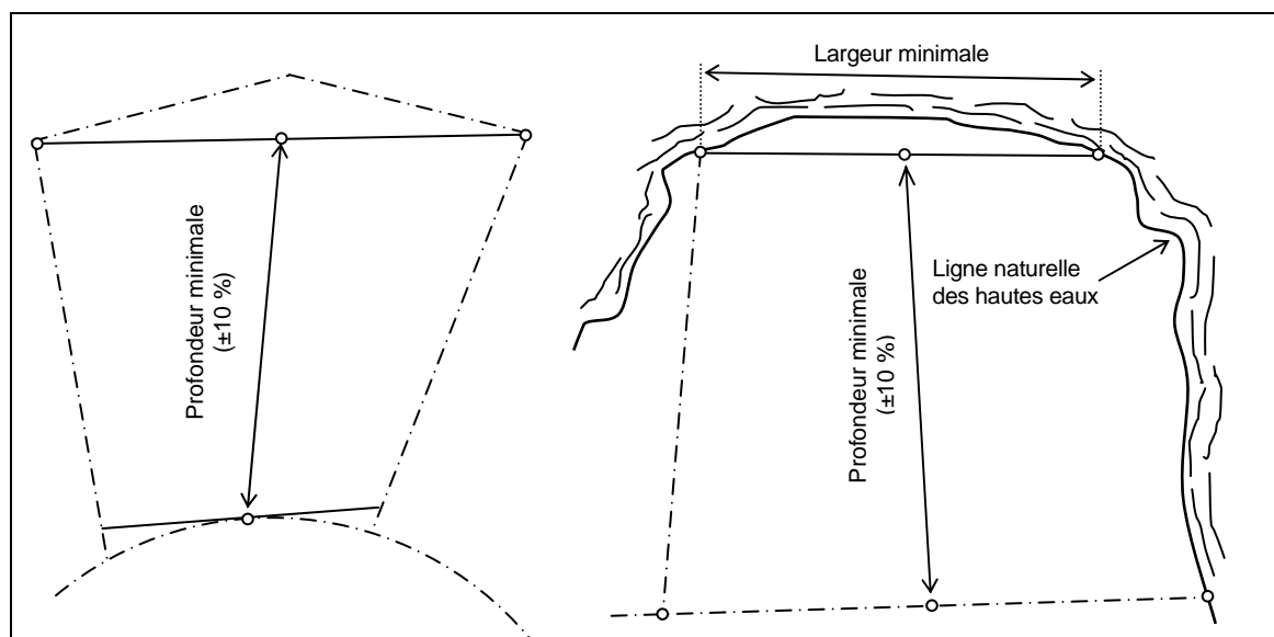
FIGURE 3.1 : CALCUL DE LA PROFONDEUR MINIMALE D'UN LOT IRRÉGULIER OU RIVERAIN
